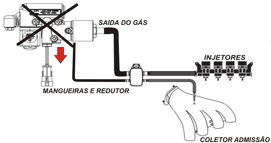
MONTAGEM INCORRETA
