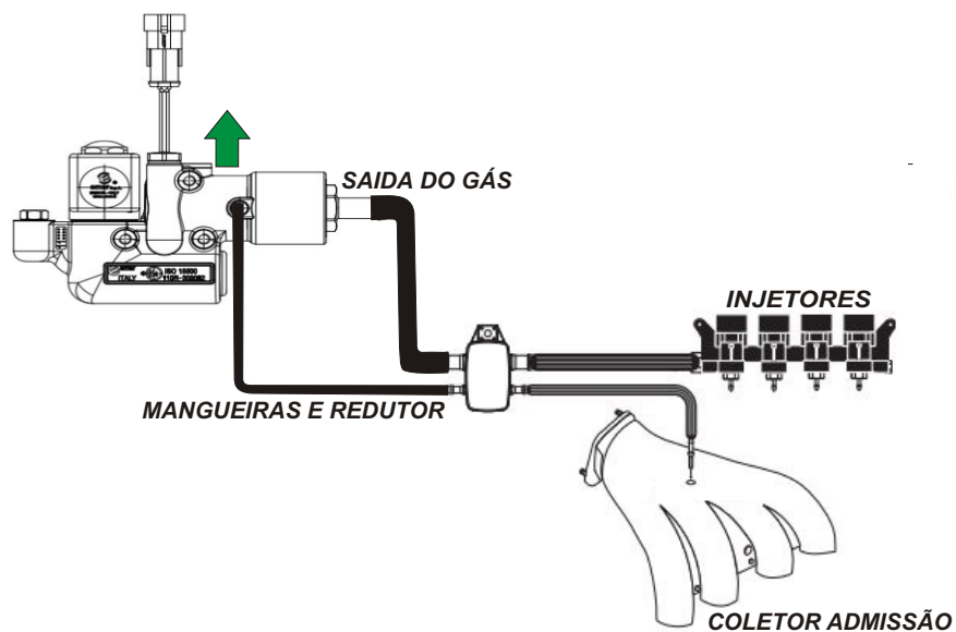
MONTAGEM CORRETA
