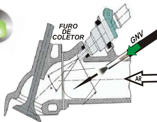
MONTAGEM CORRETA
