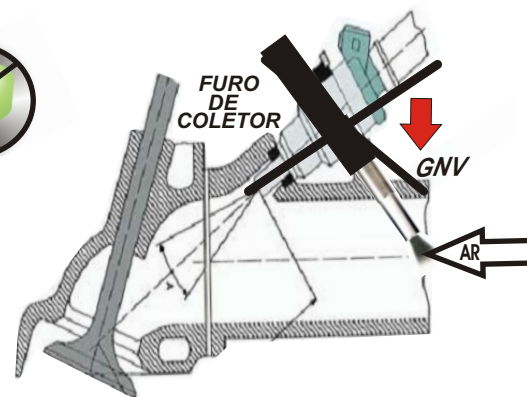
MONTAGEM INCORRETA
